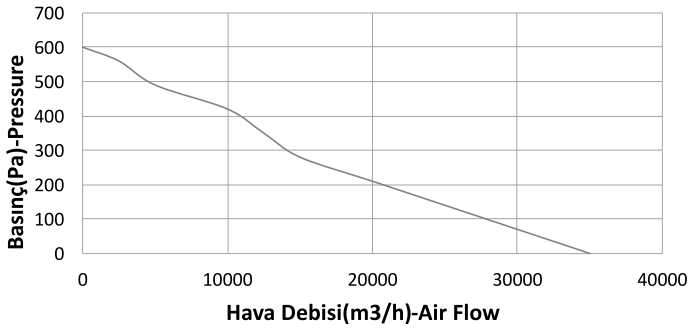
G900 - 11 kw
